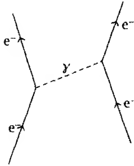
شكل ٩-١٥: يتداخل إلكترونان بتبادل فوتون.
